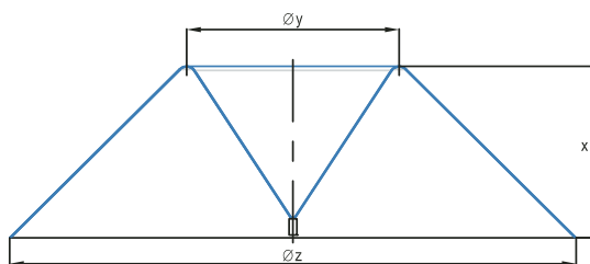
WP 3: Efecto de agua Screen Jet wide La boquilla crea una película de agua transparente.
