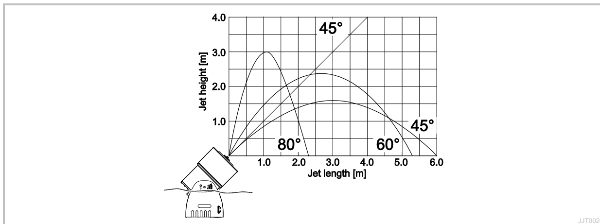
Chorro de agua con un ángulo de inclinación de 45° y en dependencia del caudal de paso y la presión del agua
